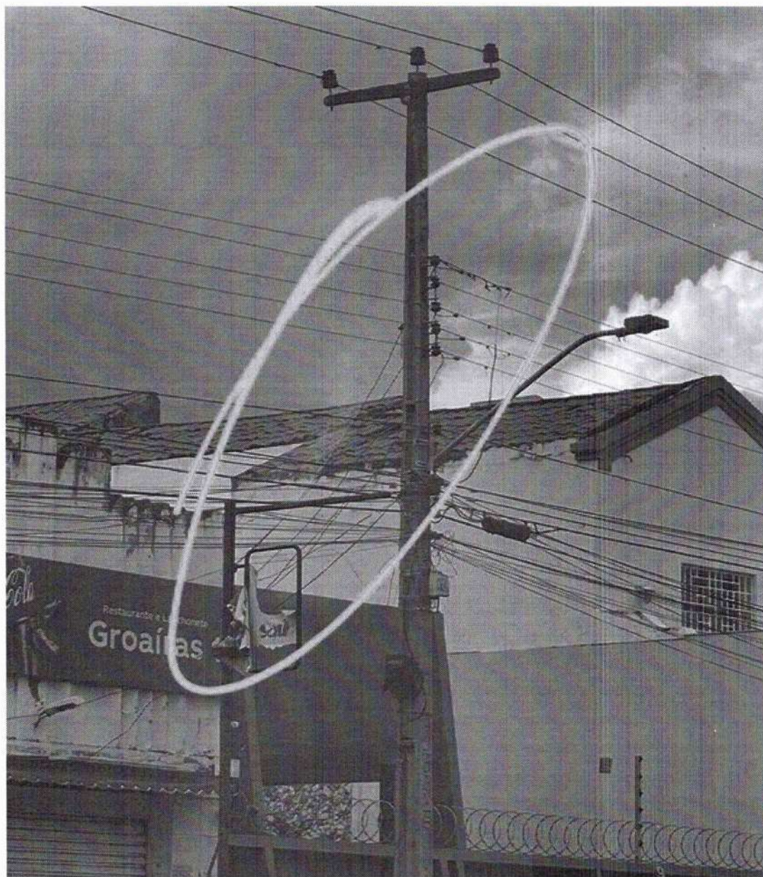
Figura 37 - Imagens de terceiros obtidas de vídeos realizados no dia do incêndio mostram um cabo de energia à aproximadamente 30m do prédio sinistrado, apresentando sinais de superaquecimento, caracterizado por emissão de fumaça.
