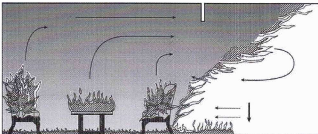
Figura 4 - Ilustração de queima generalizada( flashover ) em um cômodo. Fonte: Adaptado de NFPA 921/2014 Guide for Fire and Explosion Investigations.
