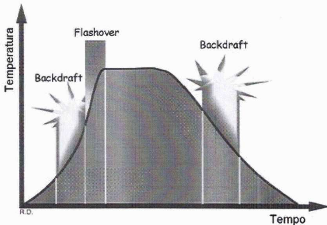
Figura 6 - Ilustração da curva dos fenômenos extremos do fogo confrontando com as fases de um incêndio.
